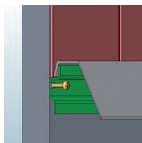
2 tasseaux métalliques d'installation baignoire
